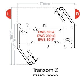
Transom Z EWS 7003
